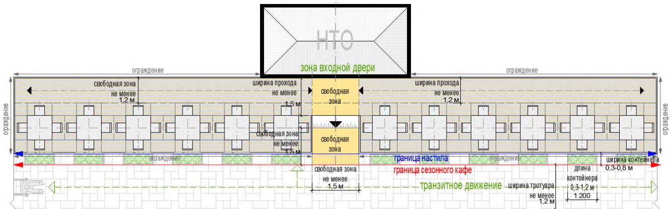
площадка сезонного (летнего) кафе 26-50 мест с павильоном или блоком модулей палаток и технологическим настилом, двухрядное размещение:
