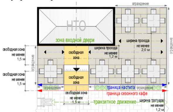
площадка сезонного (летнего) кафе 26-50 мест с павильоном или блоком модулей палаток и технологическим настилом, однорядное размещение:
